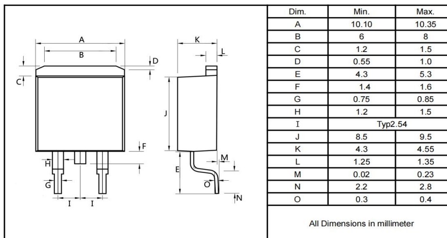
TO-263
